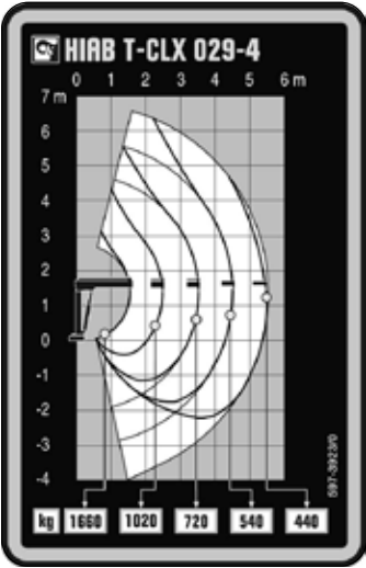
Load diagram HIAB T-HIDUO 029-4
